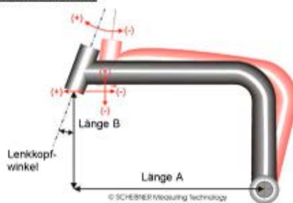
Ansicht: seitwärts
